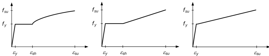
【그림 7.3】 철근의 강도 및 변형률
