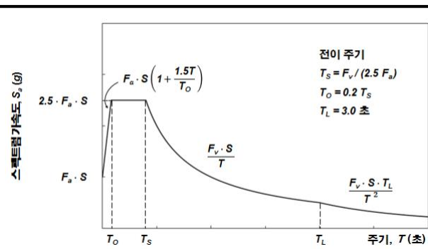
【표 9.4】가속도표준설계응답스펙트럼 (토사지반 S2~S5)
