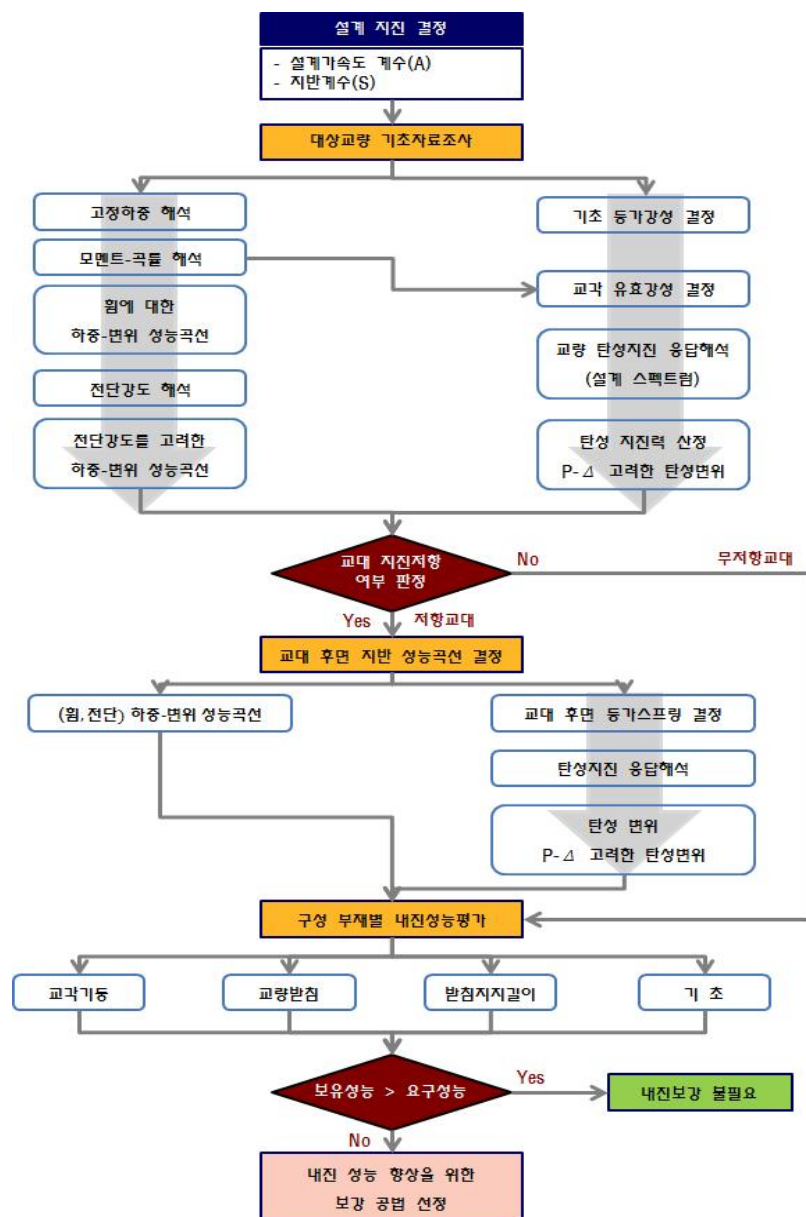
【그림 3.1】 내진성능평가 흐름도
